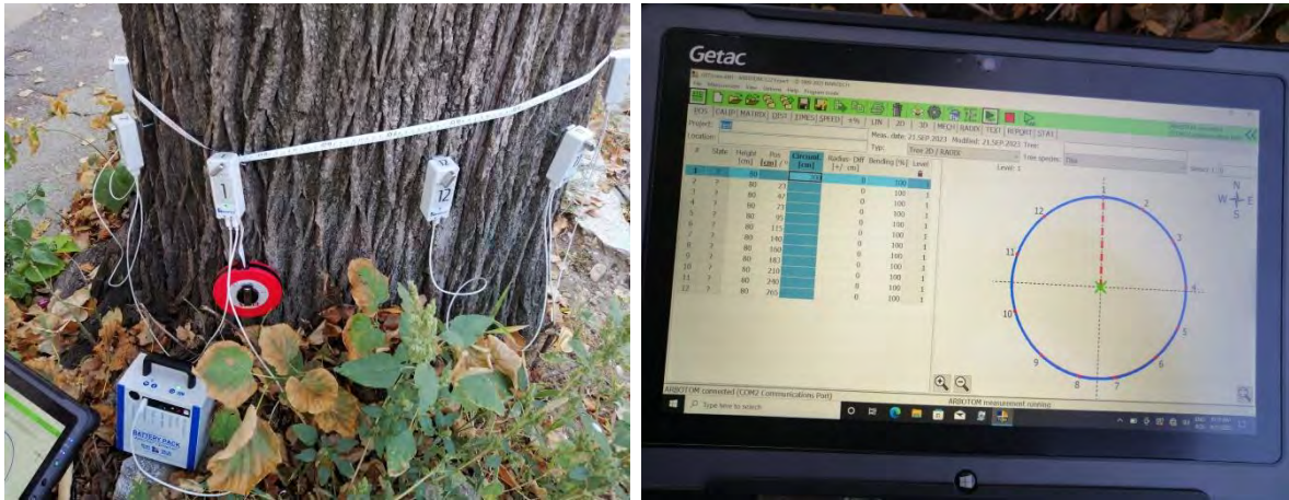
Tomograf/scanner cu ultrasunete cu 24 de senzori
